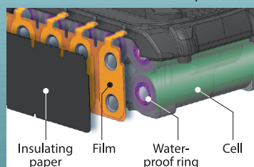
โครงสร้างสามชั้นกันน้ำ
